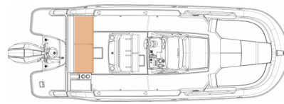
CX: 艉横巡航长条座椅
